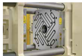
M-TECS 130 при обработке термопластов; рабочая температура – до 130°C
