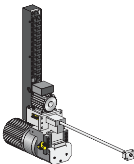
Угловой зажим с ходовым винтом
