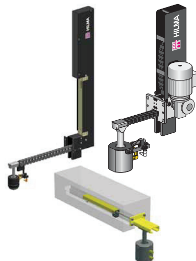
Система быстрого зажима с цепным толкателем
